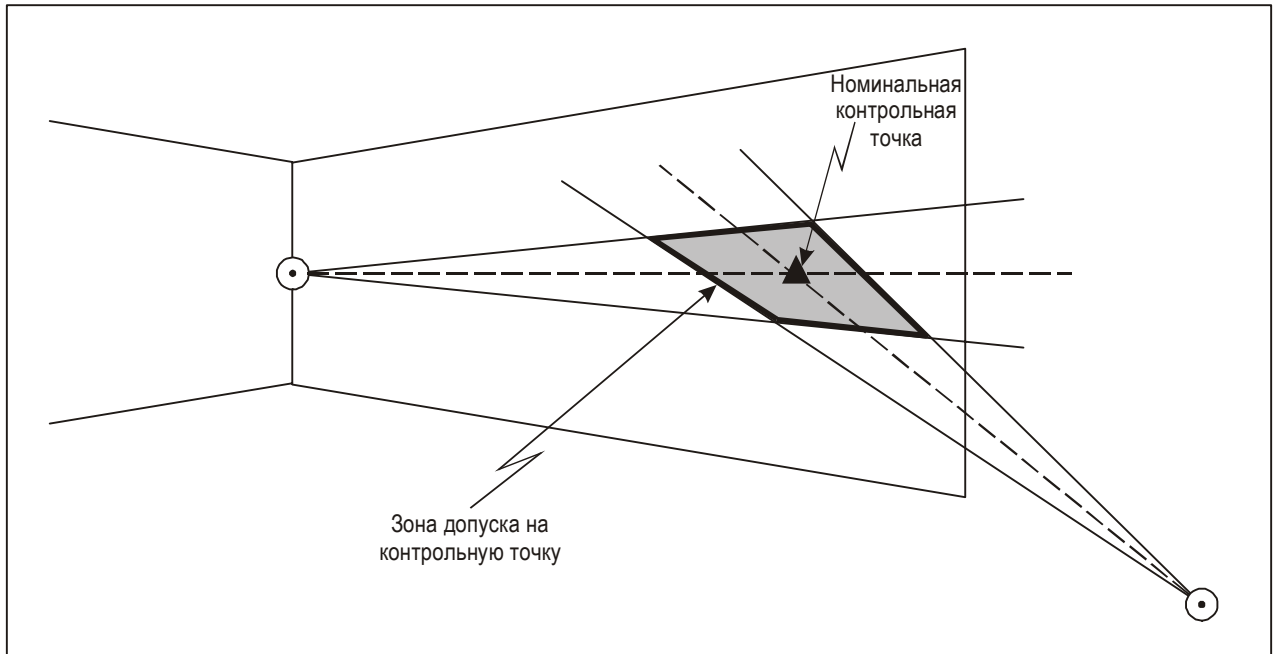
Рис. I-2-2-1. Зона допусков на контрольную точку
