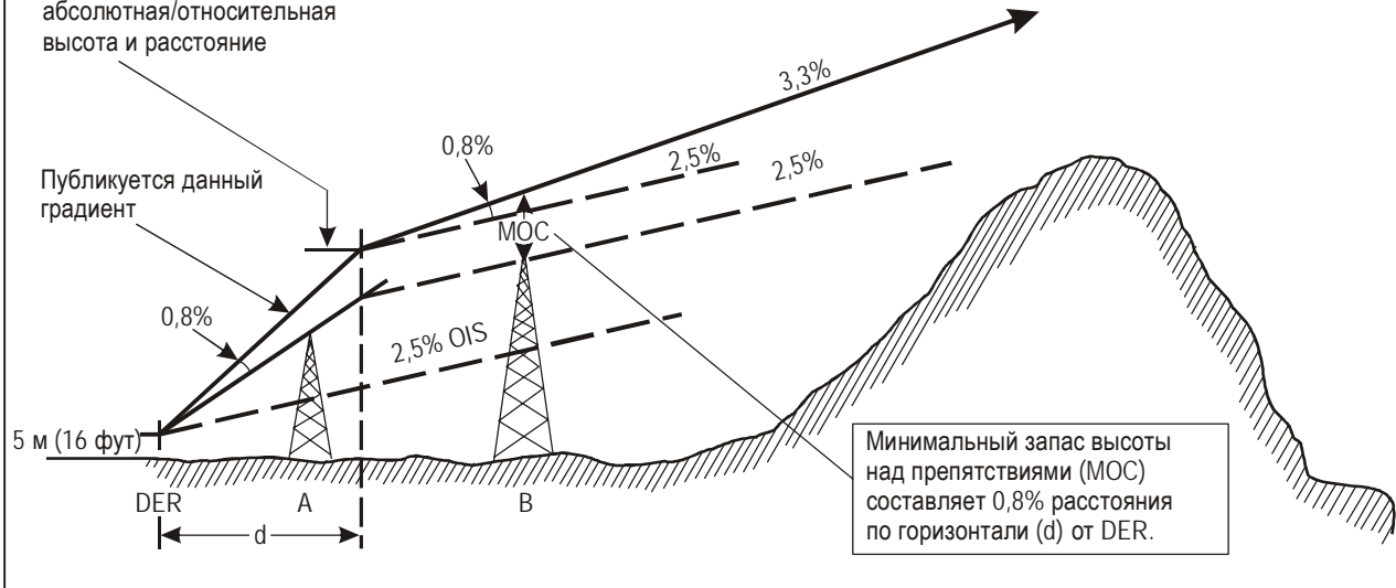
Рис. I-3-1-2. Уменьшение градиента набора высоты при вылете
