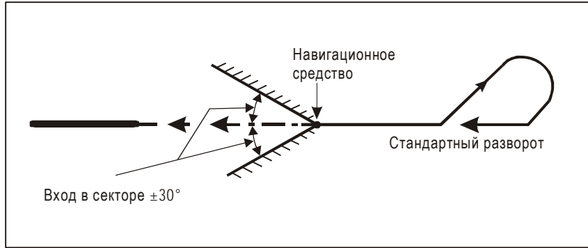
Рис. I-4-3-2. Прямой вход в стандартный разворот
