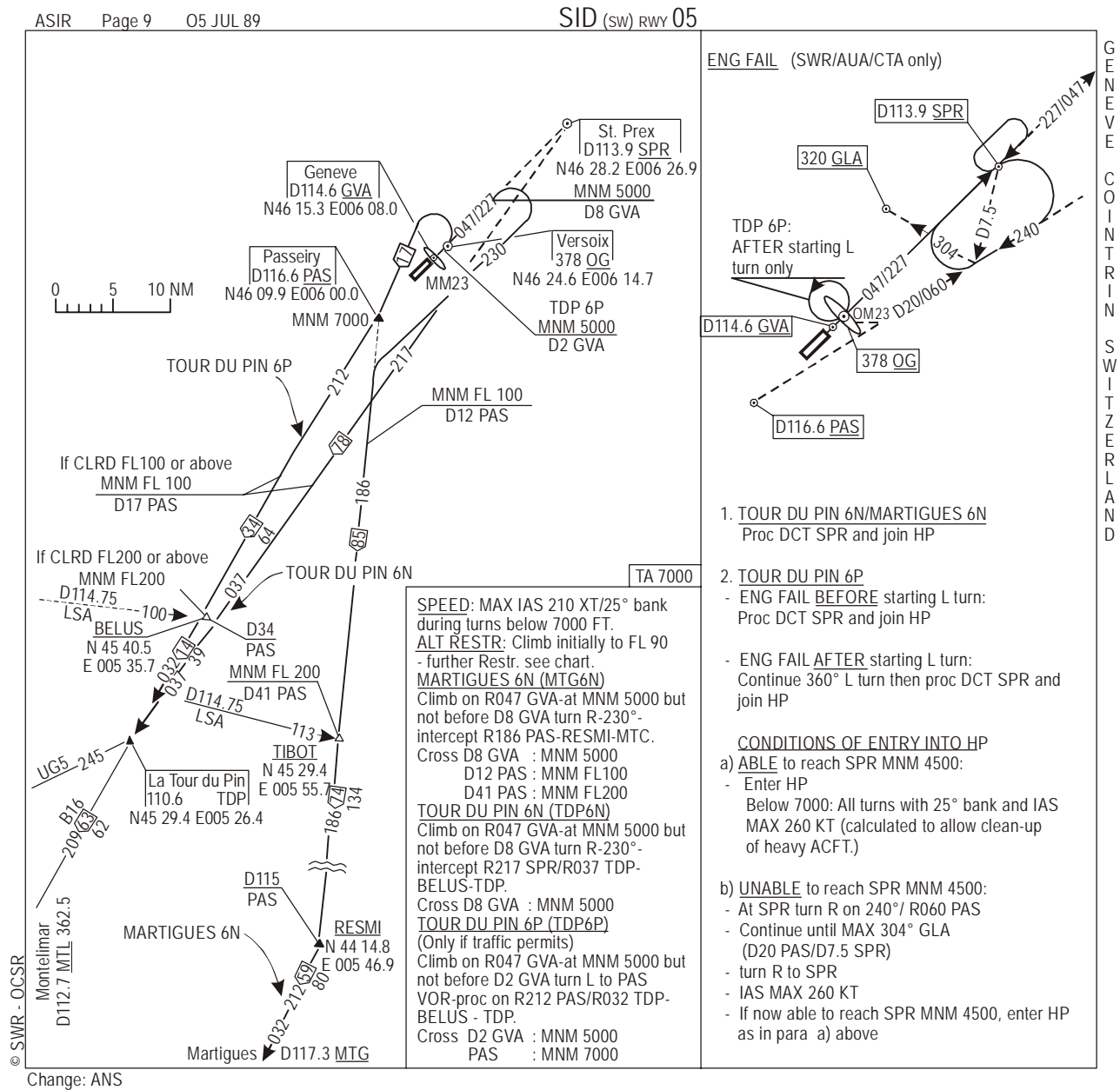
Рис. I-3-1-1. Пример запасных маршрутов в привязке к маршрутам вылета
