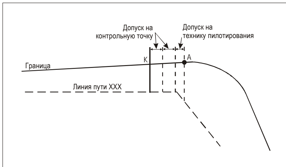
Рис. I-2-3-1. Начало построения внешней границы
