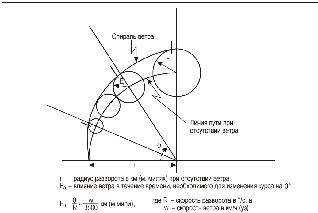
Рис. I-2-3-3. Спираль ветра
